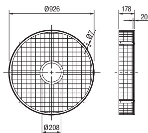
DEF 800 AN – mřížka sání (není součástí ventilátoru)
