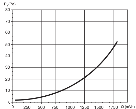
Hodnoty tlakových ztrát střešní hlavice VHO 315 v závislosti na průtoku vzduchu ve výtlačném potrubí (orientační hodnoty)
